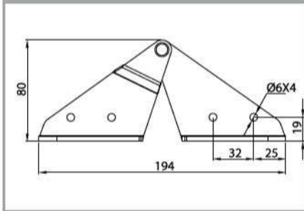
M02010416 Ürün No/Prod. No: 74 SIRT MEKANİZMA MENTEŞESİ (KALIN) BACK MECHANISM HINGE (THICK)
