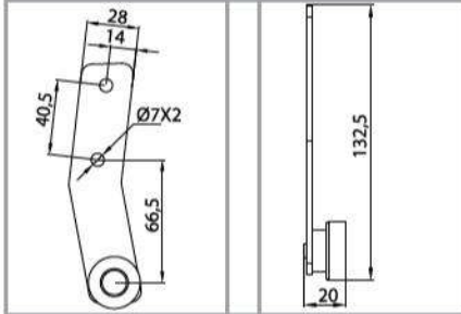
M02010280 Ürün No/Prod. No: 60 PLASTİK MAKARA TAKIMI PLASTIC BLOCK-TACKLE SET
