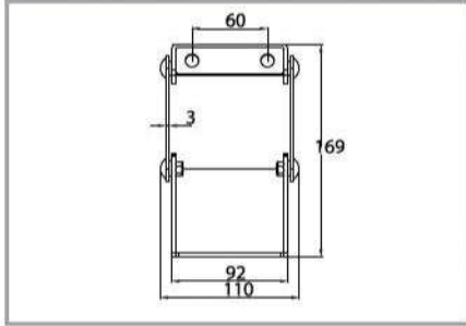
M02010411 Ürün No/Prod. No: 7 SIRT HAREKET MEKANİZMASI BACK MOTION MECHANISM
